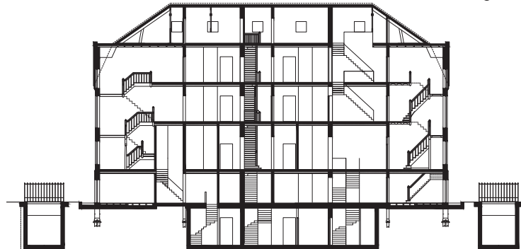
doorsnede
