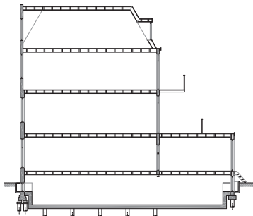
doorsnede
