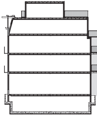
doorsnede
