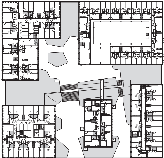
plattegrond
