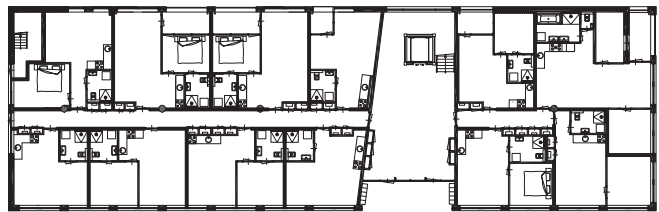
begane grond
