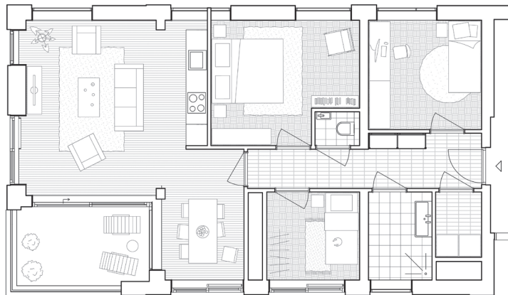
plattegrond woningtype 2
