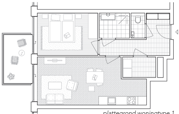
plattegrond woningtype 1
