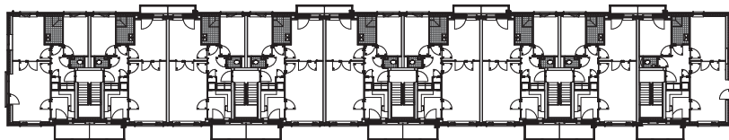
eerste verdieping
