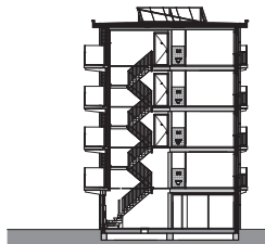
doorsnede
