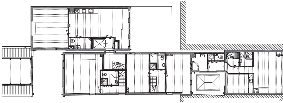
tweede verdieping
