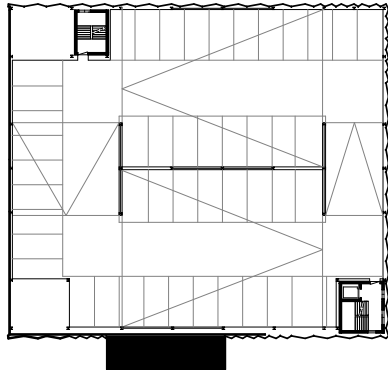
plattegrond parkeerverdieping
