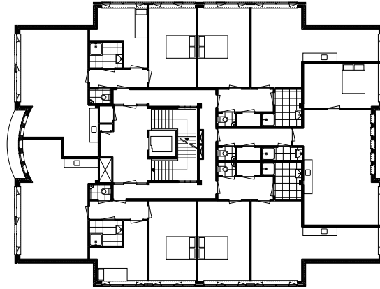
eerste verdieping
