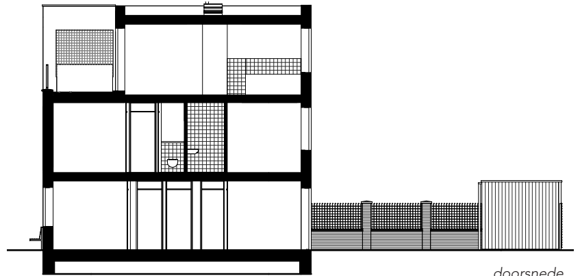
doorsnede
