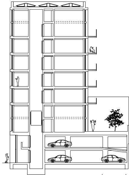
doorsnede
