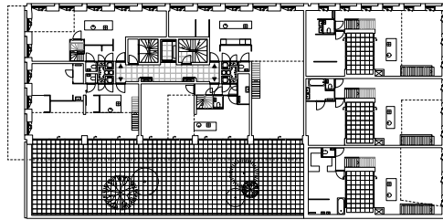
begane grond
