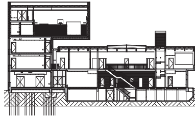
doorsnede
