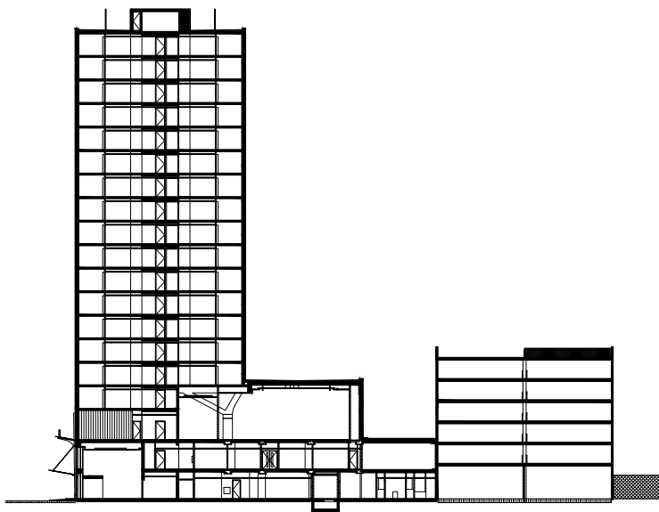
doorsnede
