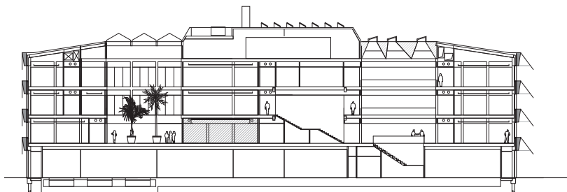
doorsnede
