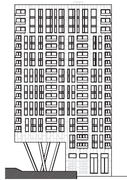
oostgevel
