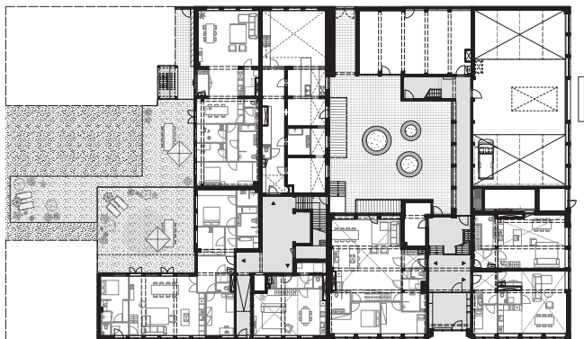
begane grond
