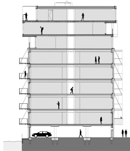
doorsnede
