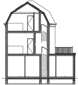
doorsnede
