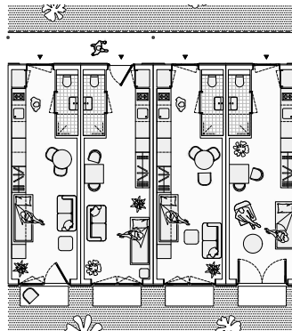
plattegrond woningen
