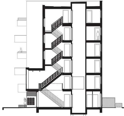
doorsnede
