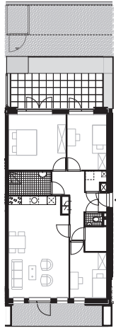
plattegrond woningtype D
