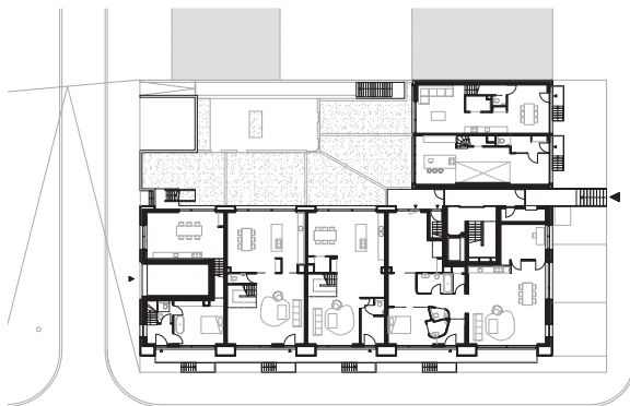
situatie met begane grond
