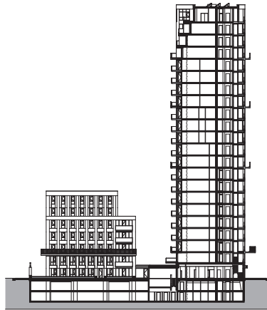
doorsnede
