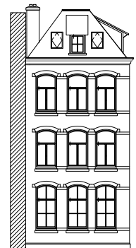
voorgevel
