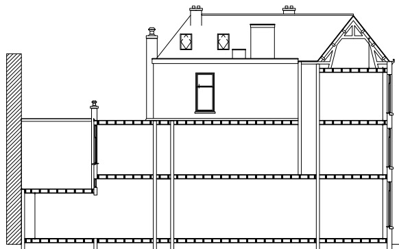
doorsnede
