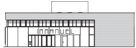
voorgevel
