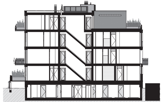
doorsnede
