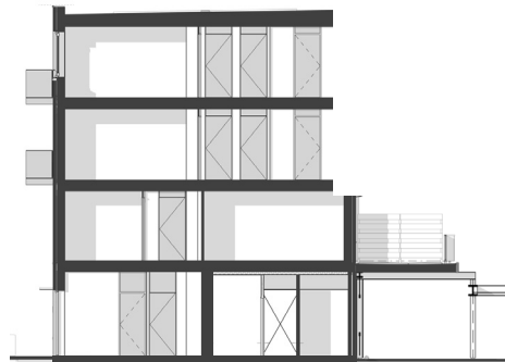
doorsnede
