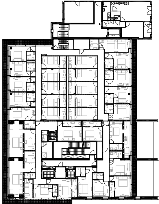
eerste verdieping
