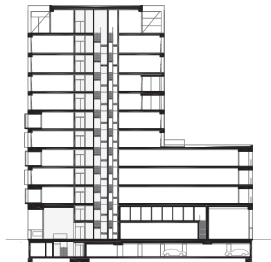
doorsnede
