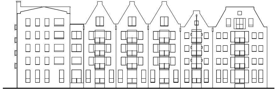
voorgevel
