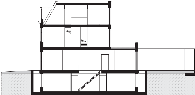
doorsnede
