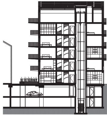
doorsnede
