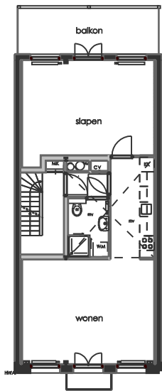
PRINCIPE PLATTEGROND
