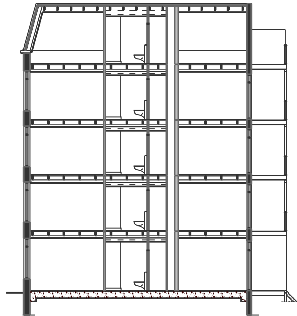
PRINCIPE DOORSNEDE
