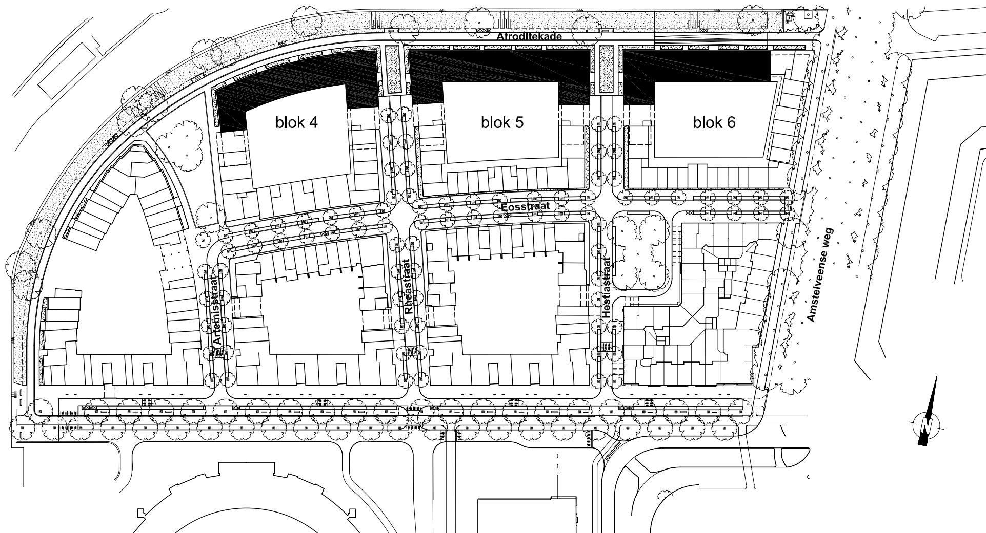
situatie Olympisch Kwartier blok 4, 5, 6
