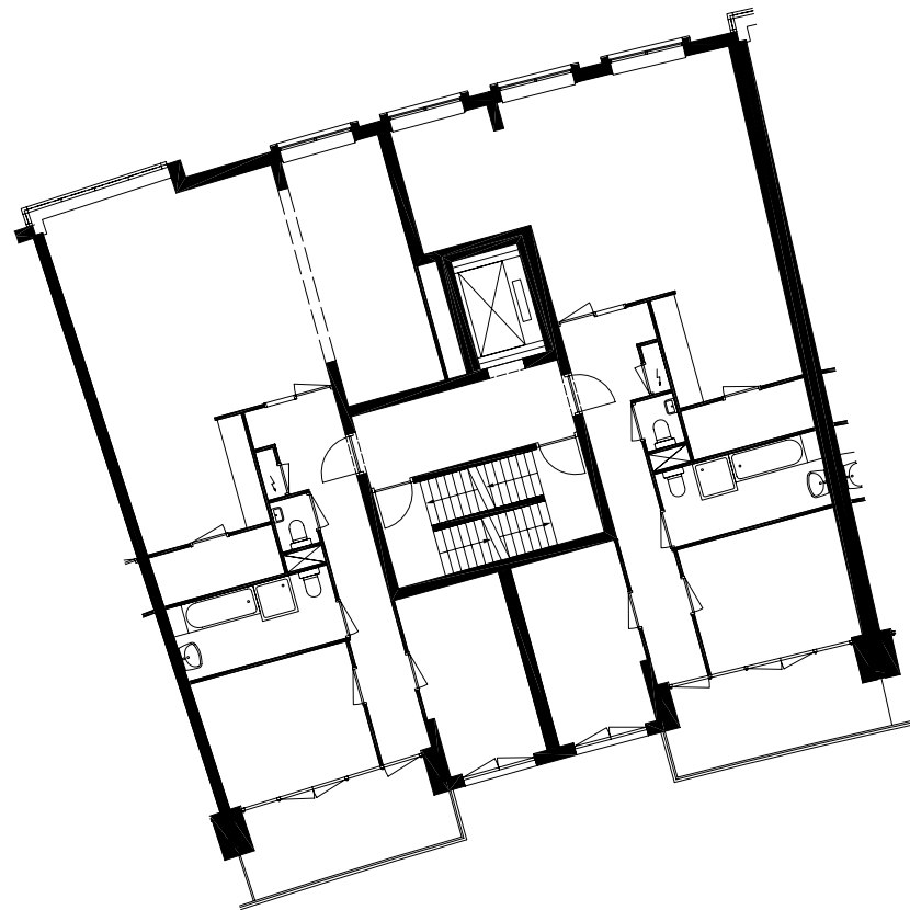
plattegrond type D2 - C6 blok 4
