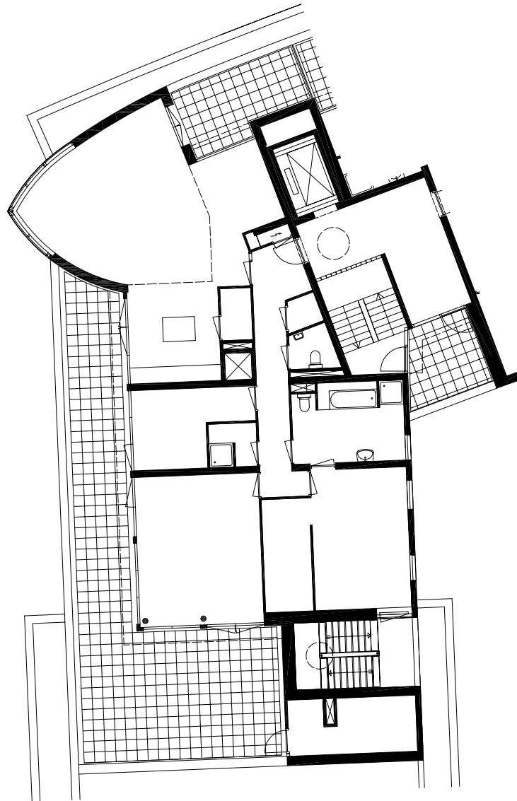
plattegrond type B3 blok 4
