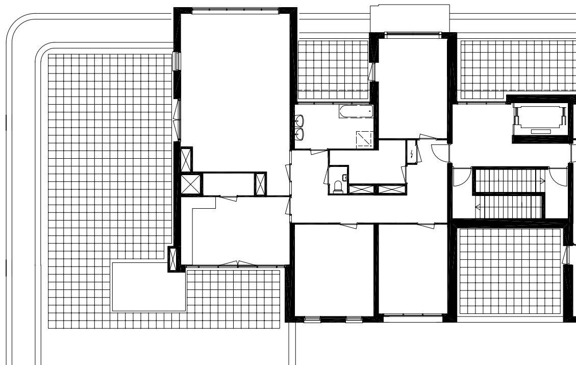
plattegrond type Koop 1 blok 6
