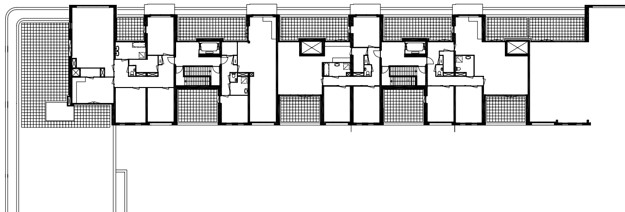
plattegrond 6e verdieping blok 6
