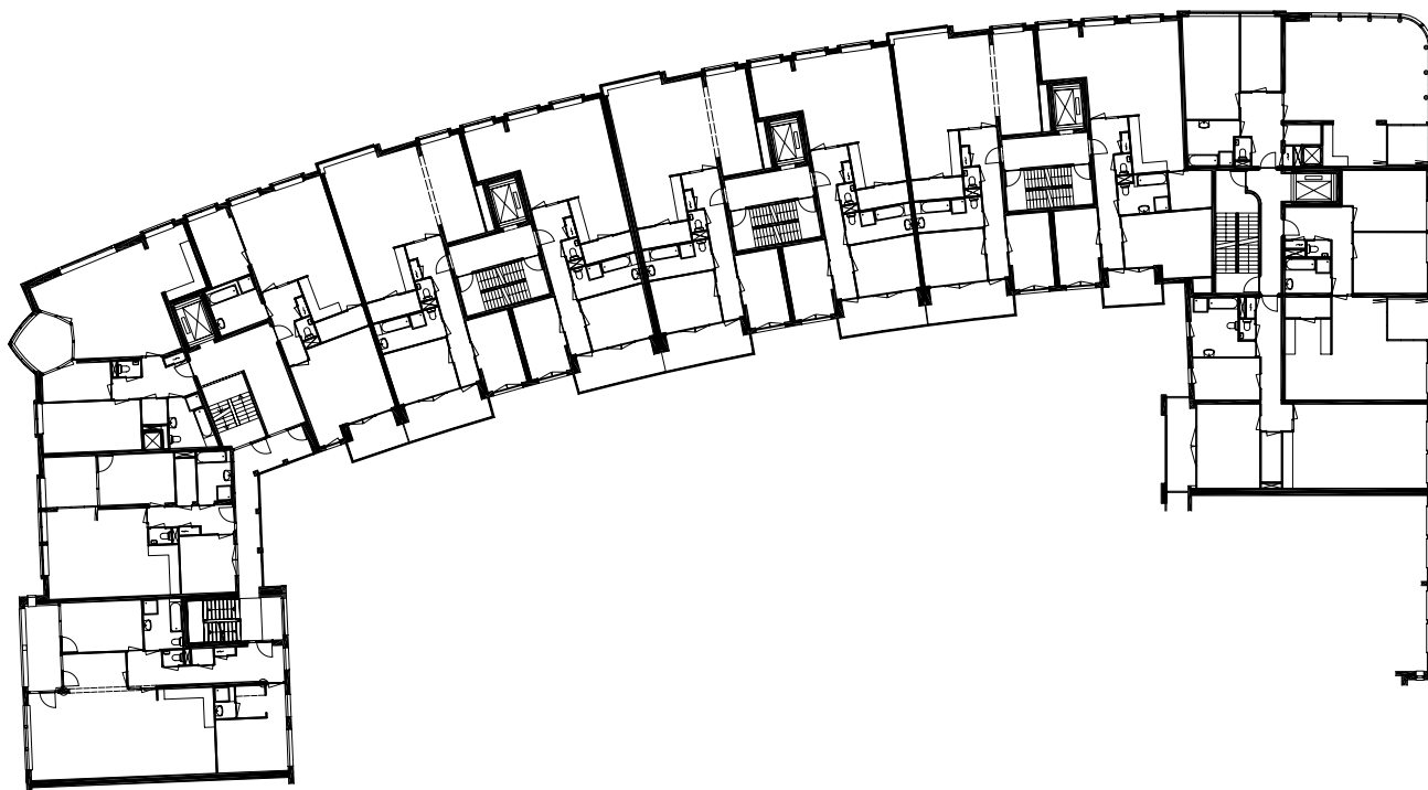
plattegrond 3e verdieping blok 4
