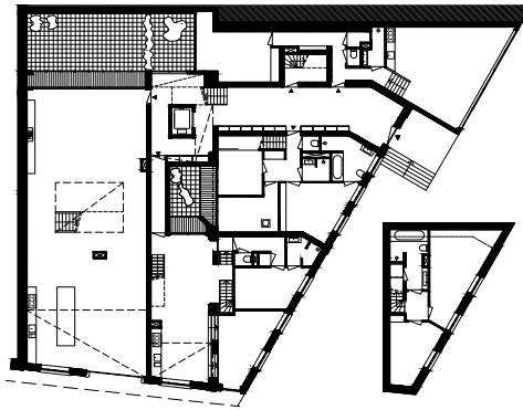
begane grond
