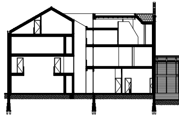
doorsnede
