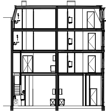
doorsnede
