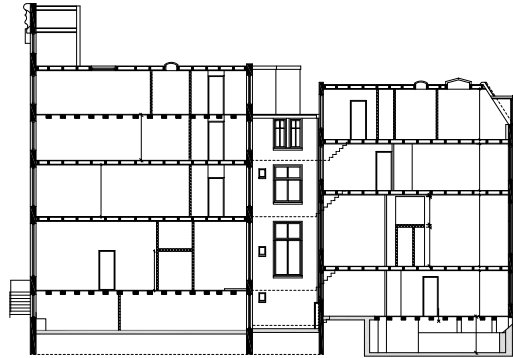
doorsnede
