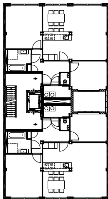
tweede verdieping
