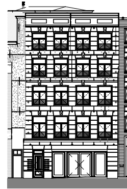
voorgevel Spuistraat
