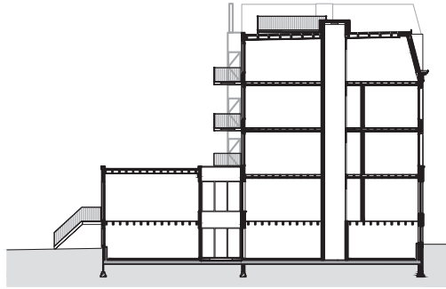
doorsnede
