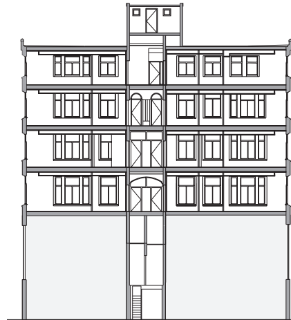
doorsnede Muntplein
