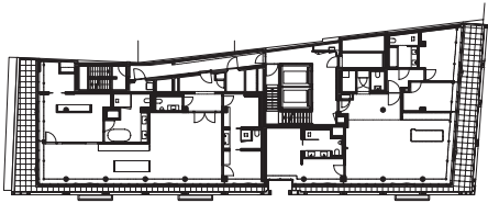
zevende verdieping
