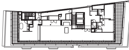
negende verdieping
