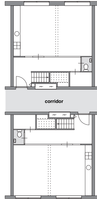
3-kamerwoning type 3kw - 1
