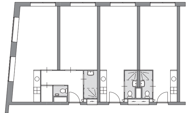
2-kamerwoning type 2kw - 1
