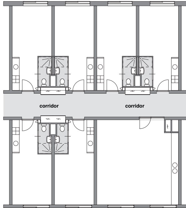
zelfstandige éénheid in groep type 1kw - 3
