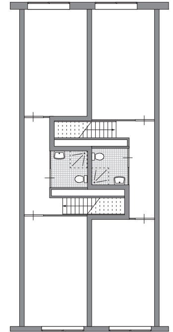
3-kamerwoning type 3kw - 1
