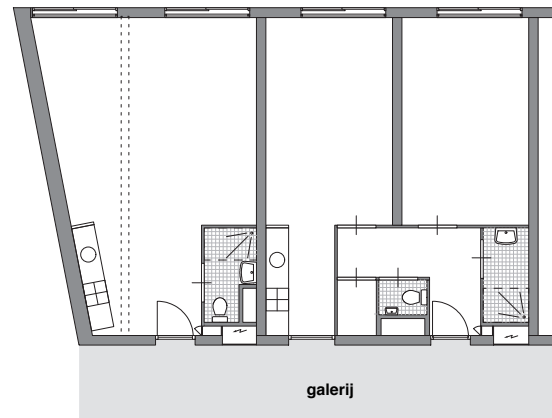
1-kamerwoning type 1kw - 2
