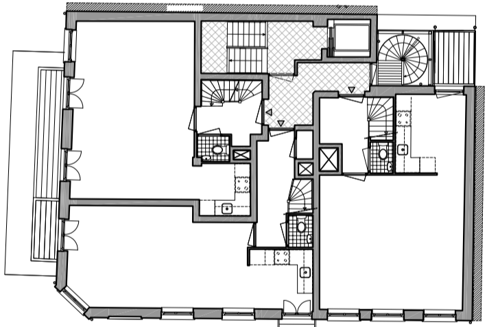
DERDE VERDIEPING
