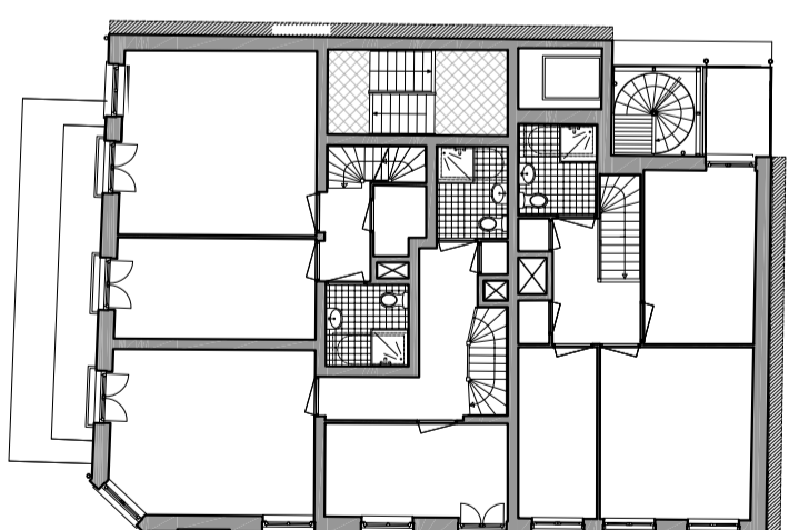
VIERDE VERDIEPING
