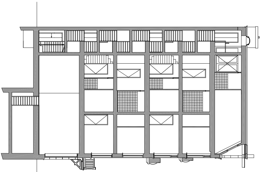
DOORSNEDE
