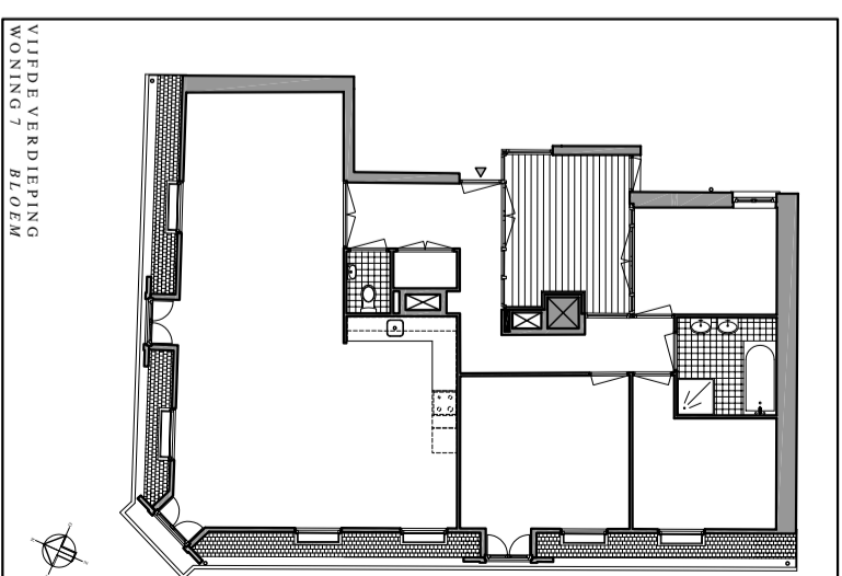
VIJFDE VERDIEPING
