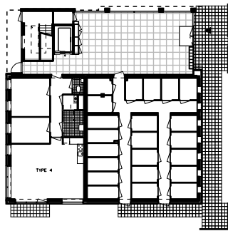
BEGANE GROND schaal 1:500
