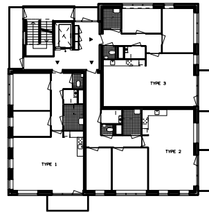
1E VERDIEPING schaal 1:500
