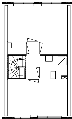
type B, 1e verdieping
