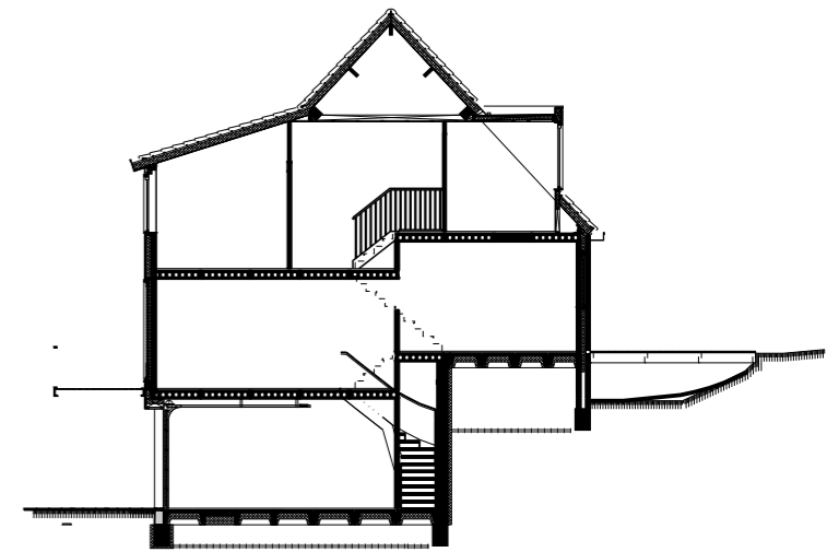
Doorsnede
