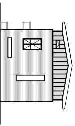
kopgevel (oost)
