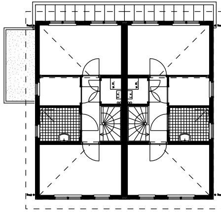
1e verdieping
