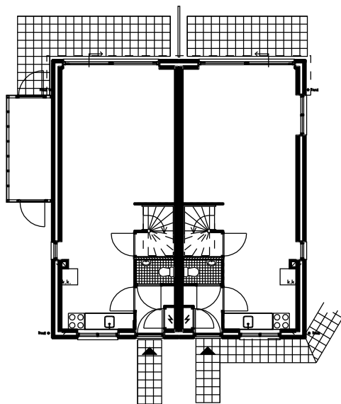
begane grond
