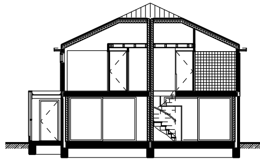
dwarsdoorsnede
