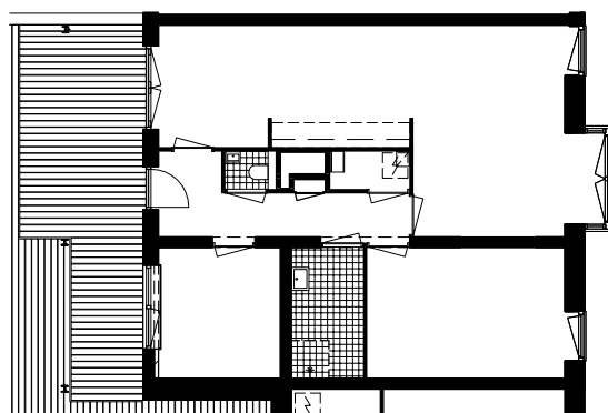
Type H2, 1e verdieping
