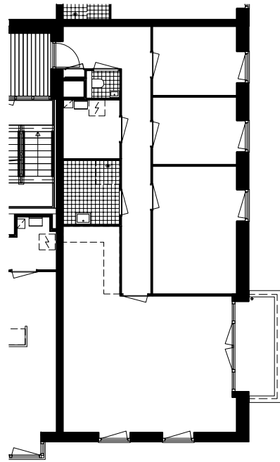
Type D1, 2e, 3e en 4e verdieping
