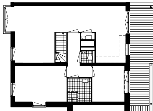
Type G, 1e verdieping
