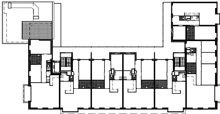
BLOKOVERZICHT 4E VERDIEPING
