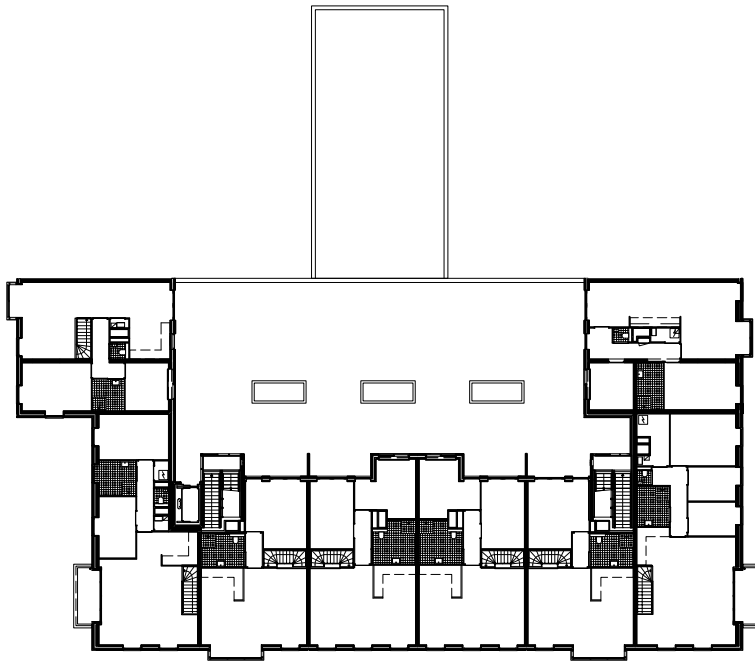
BLOKOVERZICHT 1E VERDIEPING
