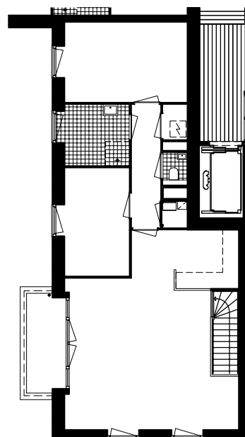
Type B, 1e verdieping
