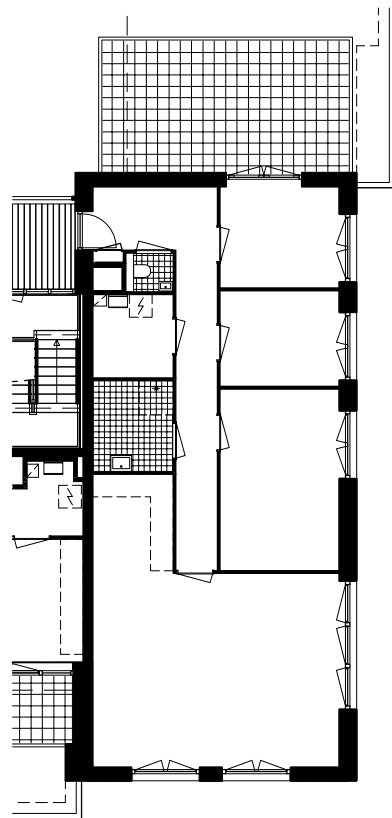
Type D3, 5e verdieping
