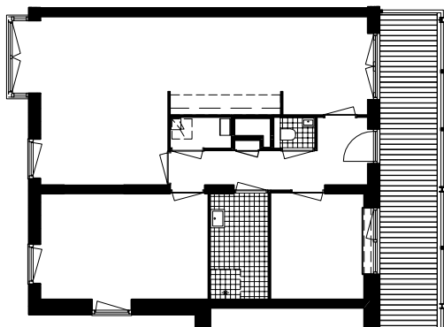
Type H, 2e en 3e verdieping
