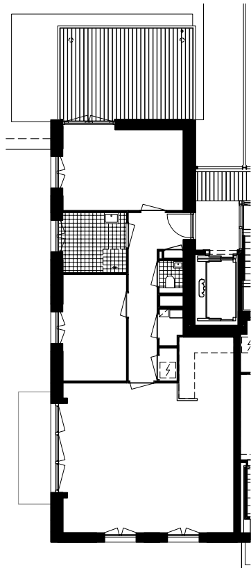
Type D2, 5e verdieping
