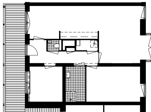
Type H1, 2e, 3e en 4e verdieping
